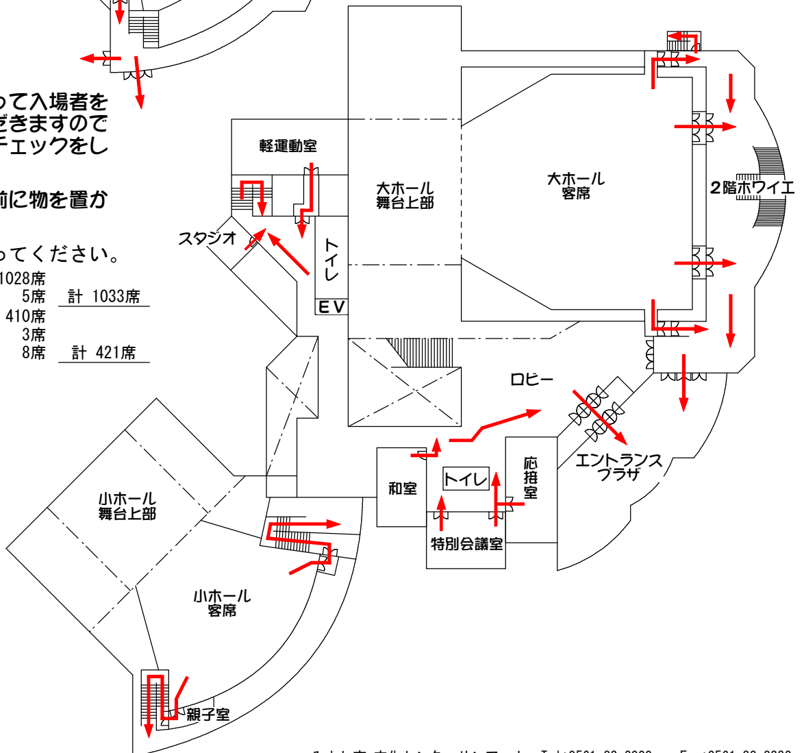
2階 平面図
